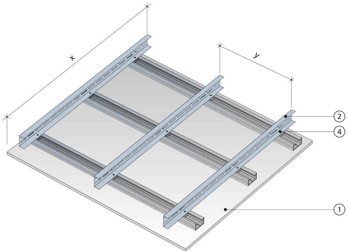
(3) Płyty gipsowo-kartonowe mocowane na konstrukcji krzyżowej dwupoziomowej z profili CD 60 i UA
