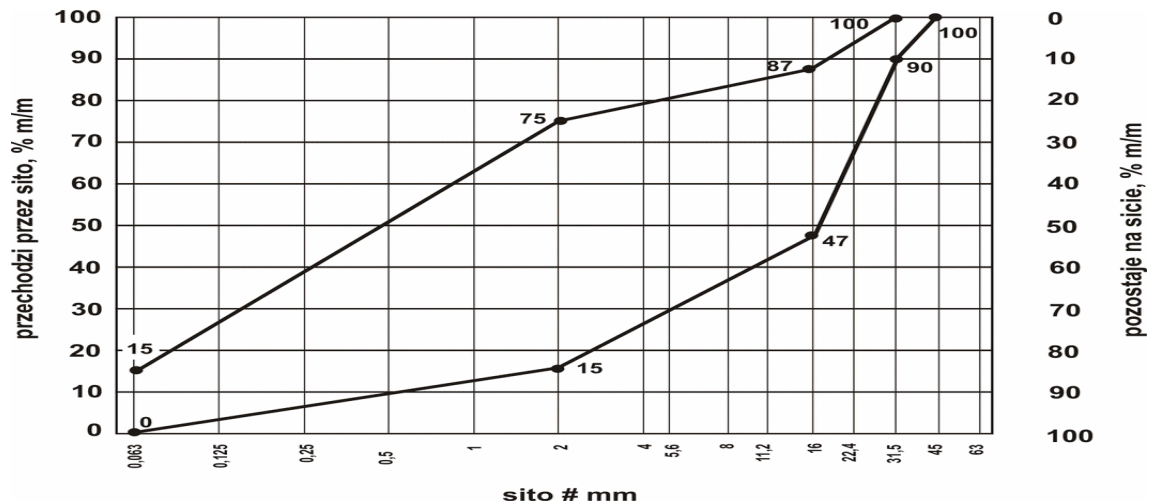
Rys. 1. Uziarnienie mieszanki niezwiązanej 0/31,5 dla warstwy mrozochronnej
