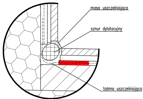
szczegół A
